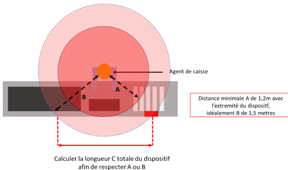
Fig2 : Meuble de caisse vue de hauteur
